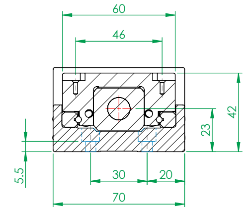
剖面圖 K-K
