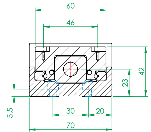
剖面圖 K-K
