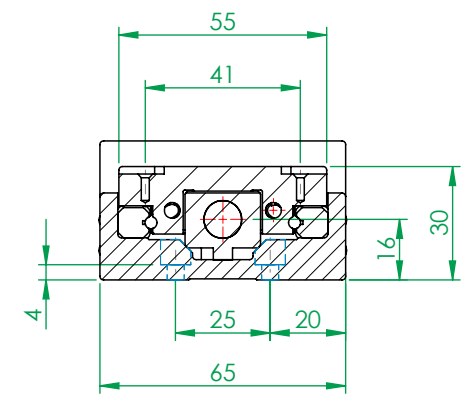
剖面圖 K-K
