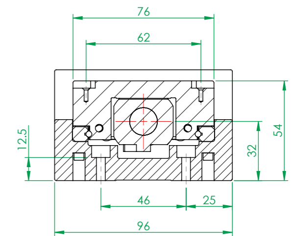
剖面圖 K-K
