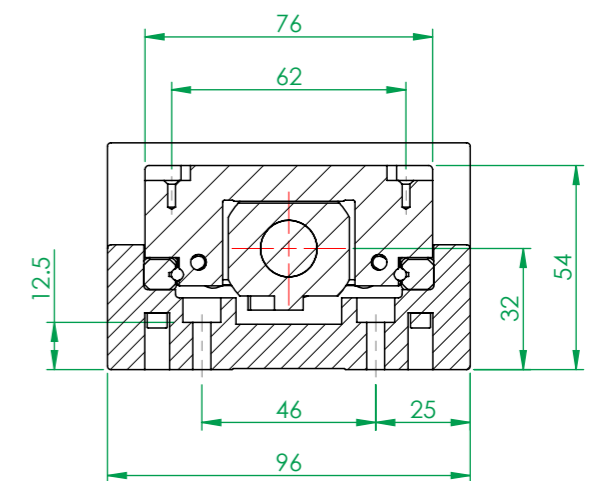
剖面圖 K-K
